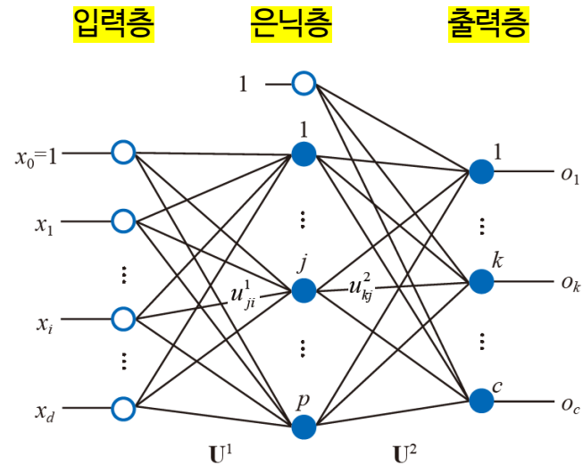
그림 4-13 다층 퍼셉트론의 구조
